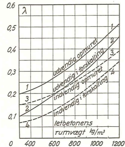
Fig. 3. Varmeledningstal for letbeton i blokke eller plader.
